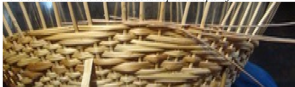
Obr. 46: Presne naproti veľkému uchu si označím miesto a tam začínam rýmovku založením 4-och prútov tenkými koncami a pletiem ťahom „cez 3 za 1“.
