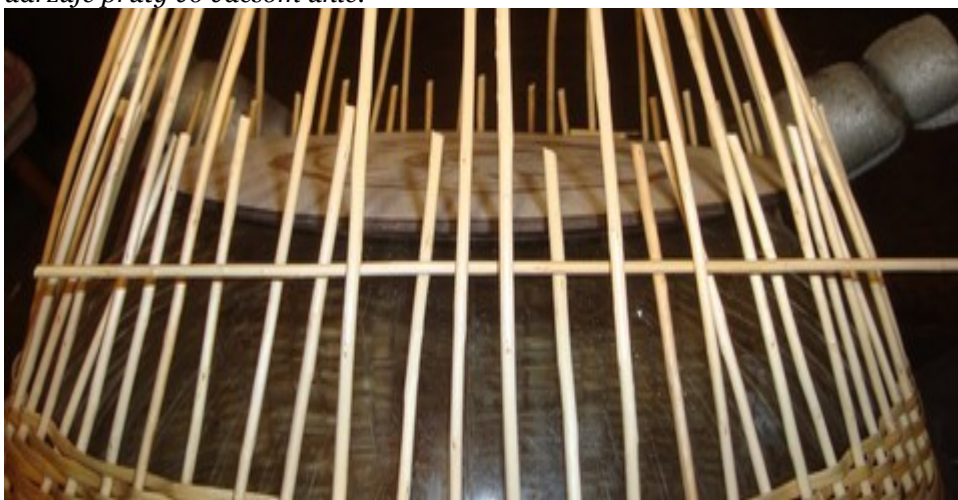
Obr. 68: Dno, ktoré má 280 mm stačí zachytiť polovičným počtom osnôv, preto každý druhý prút skrátim tak, aby prečnieval nad dnom asi 2 cm. Tým som zamedzil vzájomnému odtláčaniu prútov a lepšie sa mi bude výplet pritláčať na sklo.
